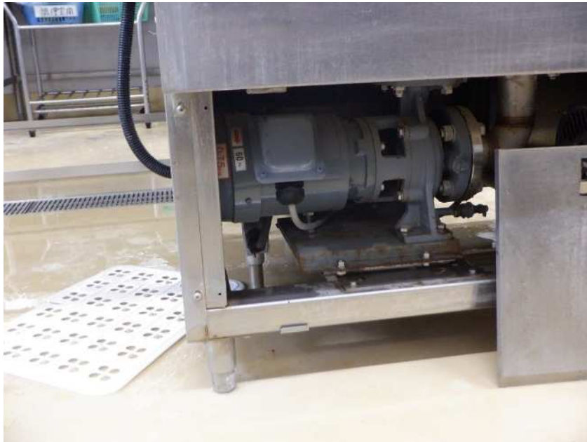
洗浄機の全長が2350mm。水栓柱及び天井扇との位置関係に配慮が必要。
