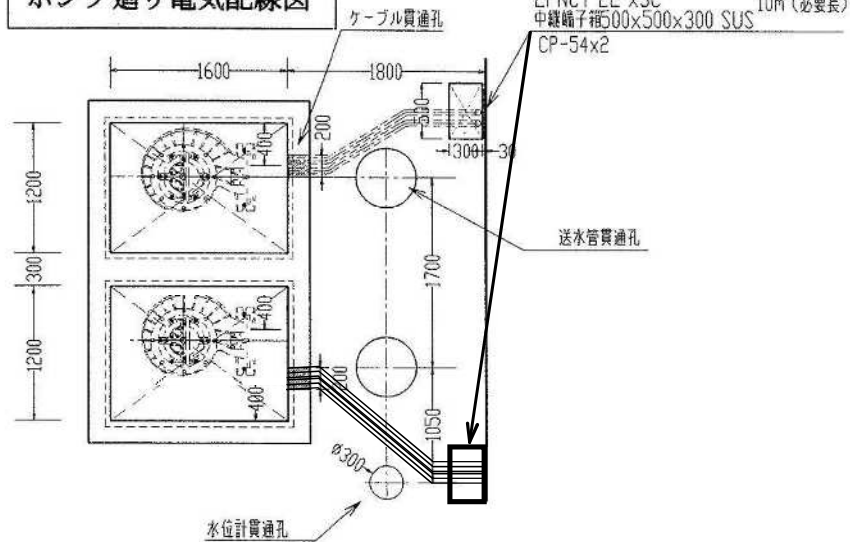
ポンプ廻り電気配線図
