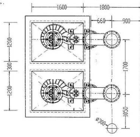
ポンプ廻り平面図
