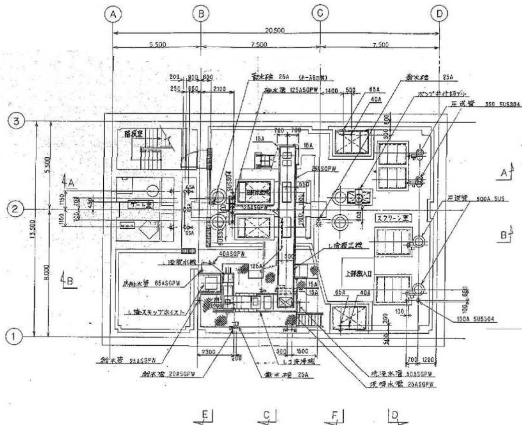
B2F (下段部) 平面図
