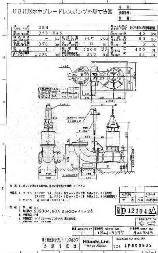
既設ポンプ図面その1
